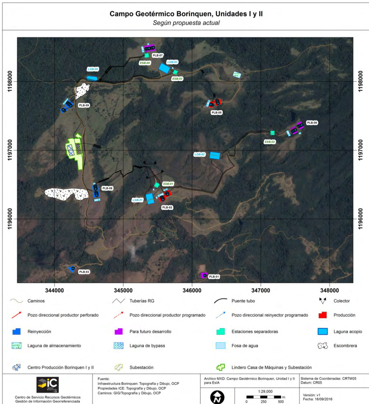
Figura 46. Sitios de obra del Proyecto Geotérmico Borinquen con modificación al diseño de obras.
